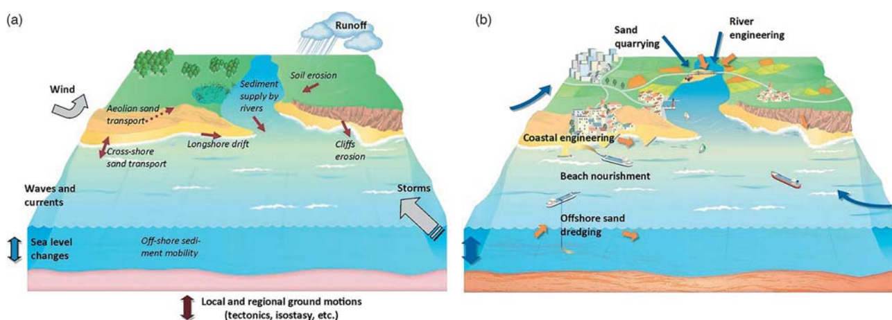
Figure 5 : Processus impliqués dans le transport des sédiments en zone côtière et l'évolution du trait de côte en l'absence d'interventions humaines (a) et sous l'influence des interventions humaines (b) d'après Cazenave et Le Cozannet (2013)
